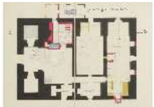
HchAS.III, Grundriss zur Schlossbrauerei Herrenwörth, DI016513, BSV
