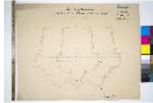
LIIMus.IV, Gurten und Wölbrücken, Profil, Palas, 3. OG, Neusch., DI031313, BSV-
