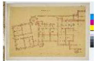
LIIMus.IV, Grundriss Palas, 1. OG, Neusch., DI030947, BSV-
