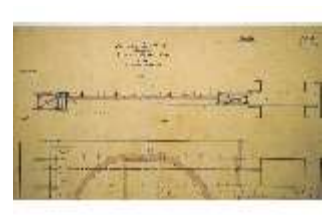
LIIMus.IV, Thronsaal, Stahlträgerkonstruktion, Ausschnitt, Neusch., DI031786, BSV-
