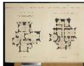
LIIMus.III,G, Grundrisse, Burg Falkenstein, 531 und 532, DI018987, BSV
