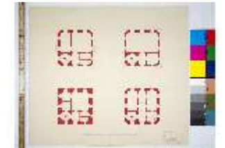
LIIMus.IV, Bergfried, Grundrisse (EG und 1.-3. OG), Neusch., DI032376, BSV-
