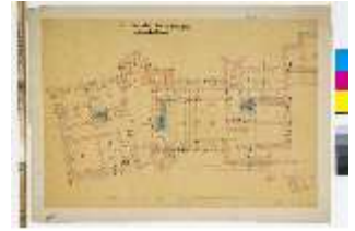
LIIMus.IV, Grundriss Palas, Parterre, Neusch., DI030933, BSV-
