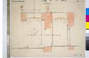
LIIMus.IV, Palas, Querschnitt der Freitreppe, Neusch., DI032188, BSV-
